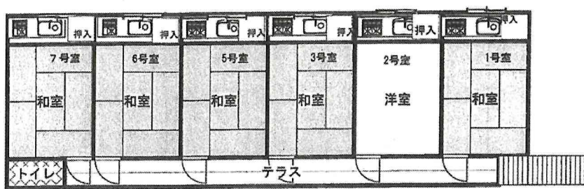
1階見取り図
